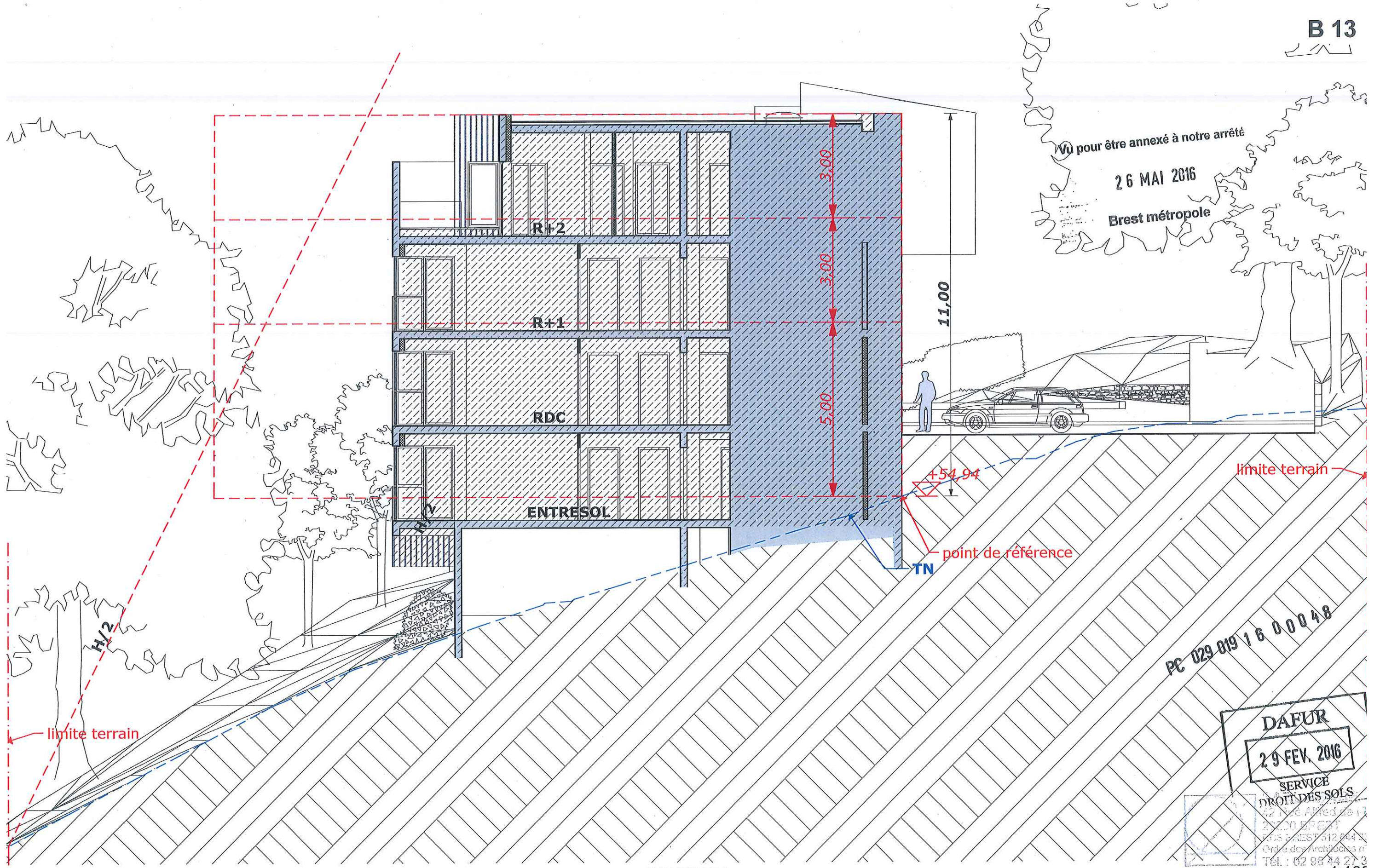
COUPE B1
